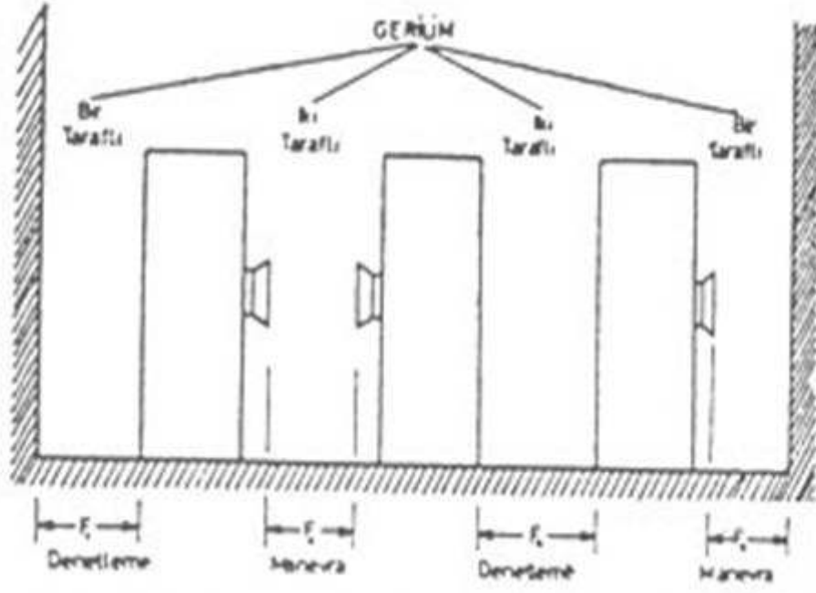
Şekil-1 Hücresel cephelerinin tel kafes kapı ve dolu duvar olması durumunda geçit genişlikleri
